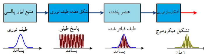
شکل ۳ طرحواره تولید شکل موج بر اساس شکل دهی طیفی نوری و نقشه برداری بسامد وابسته به زمان.
