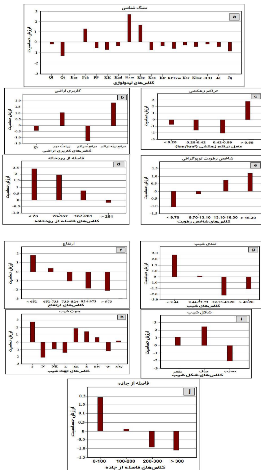
شکل ۶: ارزش حساسیت برای هر کلاس عوامل ایجاد آب‌کند: a: سنگ‌شناسی، b: کاربری اراضی، c: تراکم زهکشی، d: فاصله از رودخانه، e: شاخص رطوبت توپوگرافی، f: ارتفاع، g: تندی شیب، h: جهت شیب، i: شکل شیب، j: فاصله از جاده.
